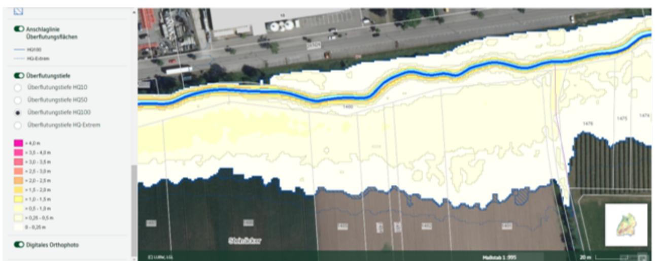
Abb. 12 Überflutungstiefen - LUBW
